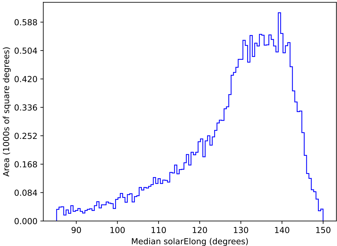
extra_ss_neo7_v3.4_10yrs All sky y band: Median solarElong
