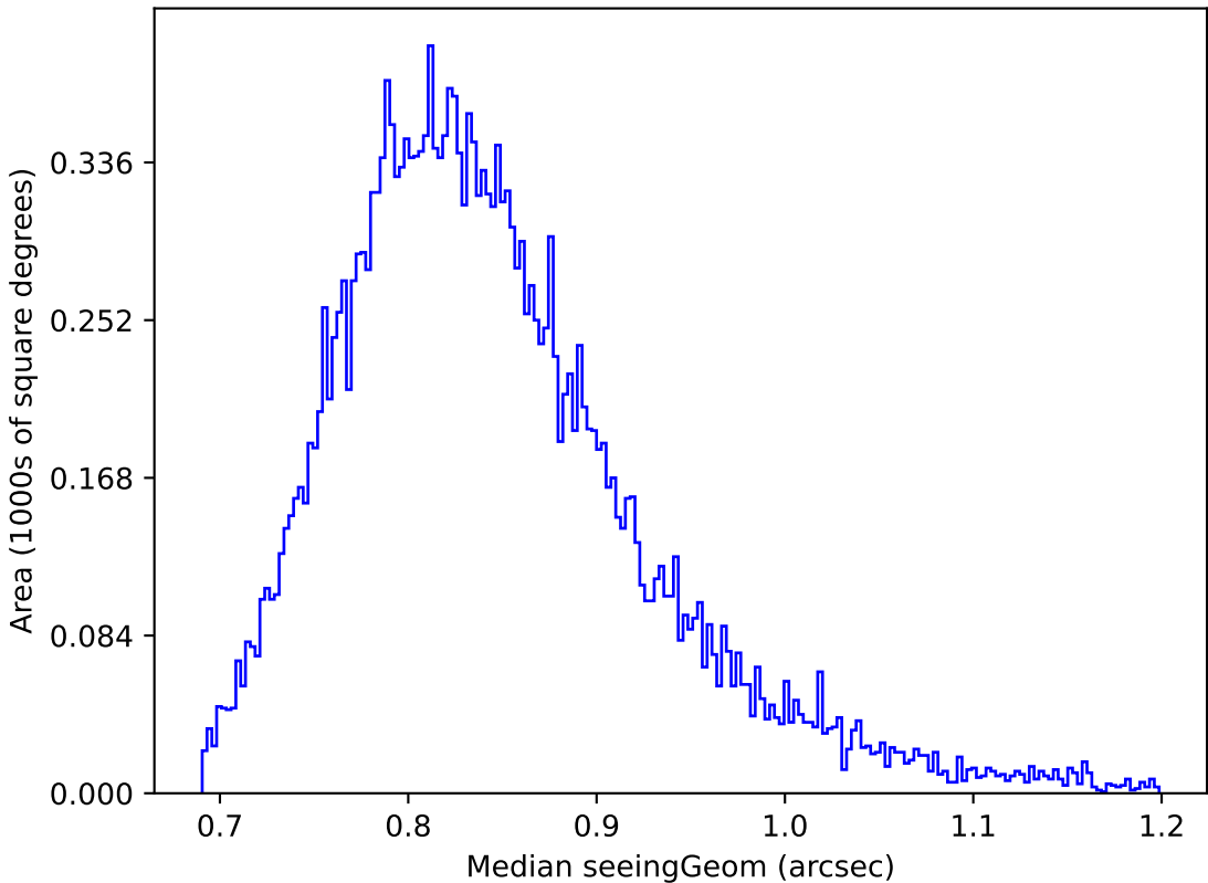
extra_ss_neo7_v3.4_10yrs Yr 1 y band: Median seeingGeom
