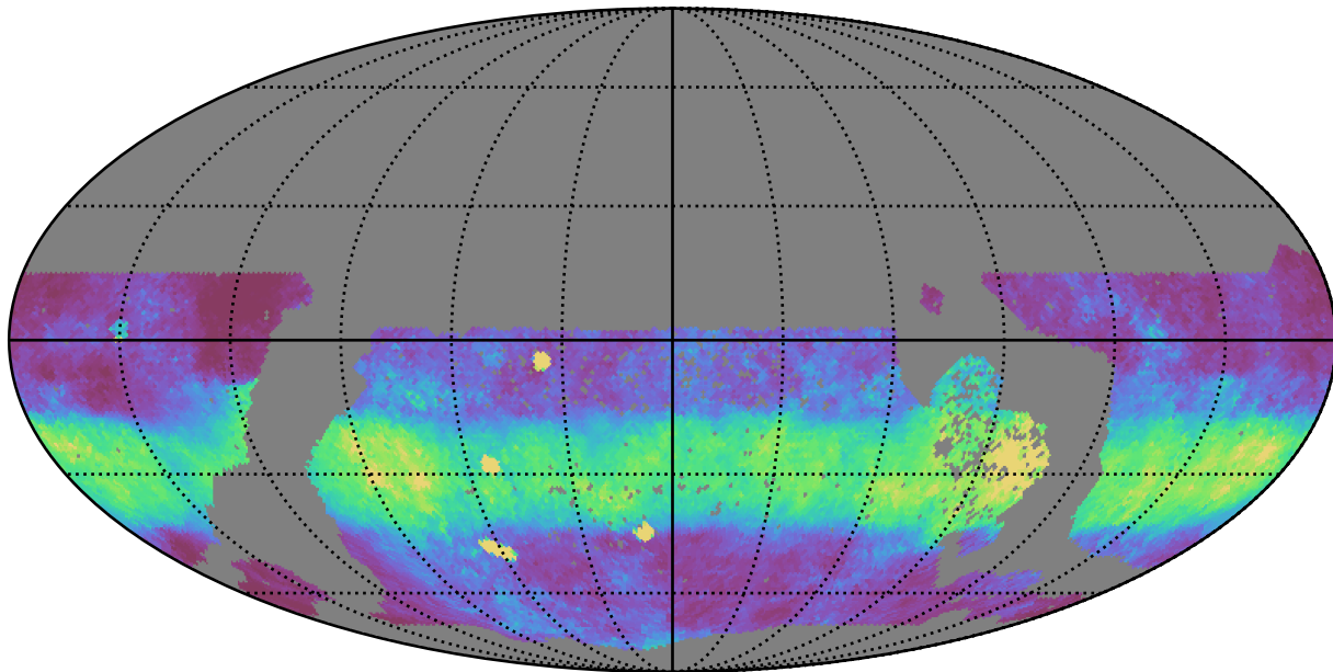
extra_ss_neo7_v3.4_10yrs WFD y band: Median normairmass
