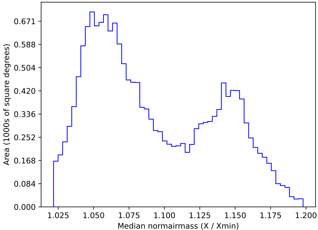
extra_ss_neo7_v3.4_10yrs WFD y band: Median normairmass
