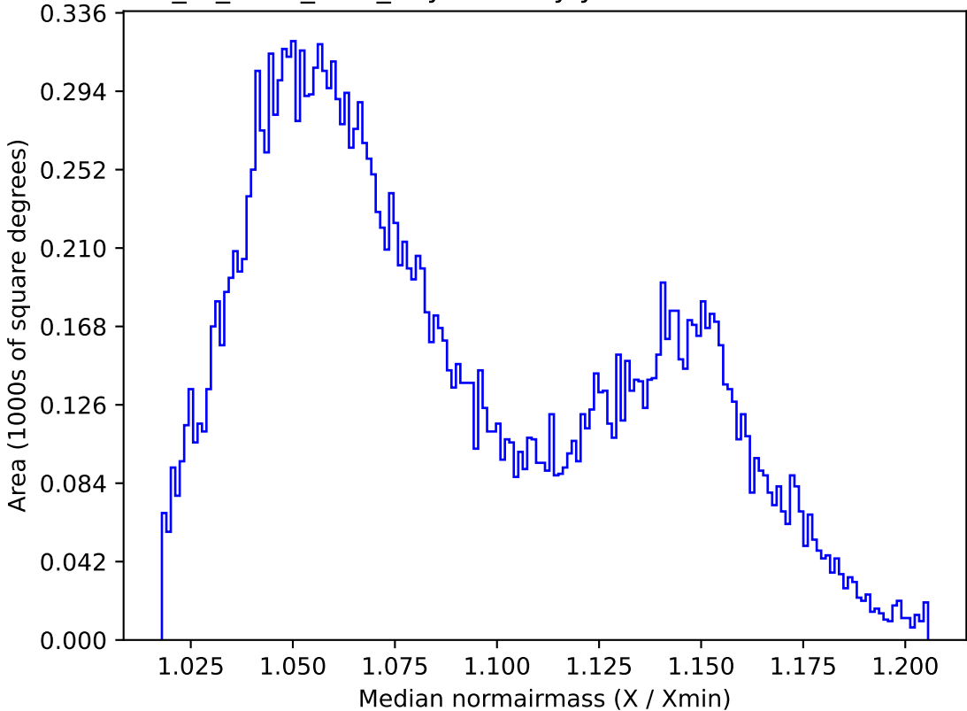
extra_ss_neo7_v3.4_10yrs All sky y band: Median normairmass
