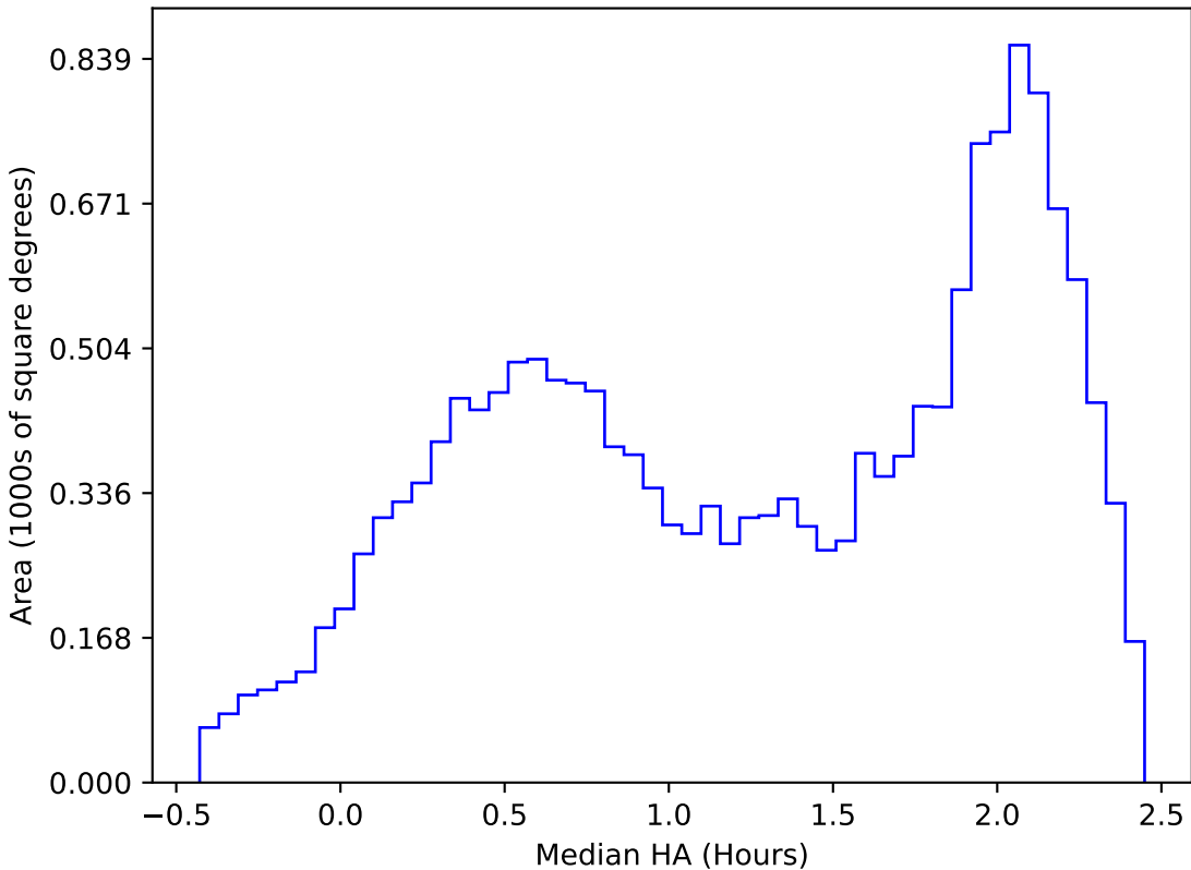
extra_ss_neo7_v3.4_10yrs WFD y band: Median HA
