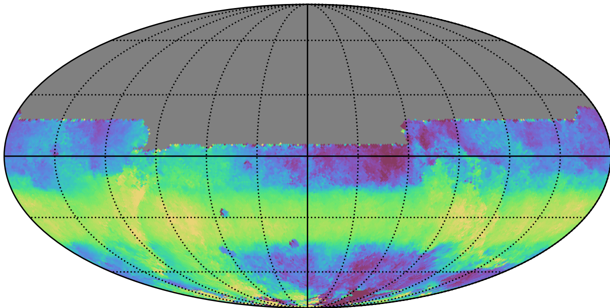
extra_ss_neo7_v3.4_10yrs All sky y band: Median HA
