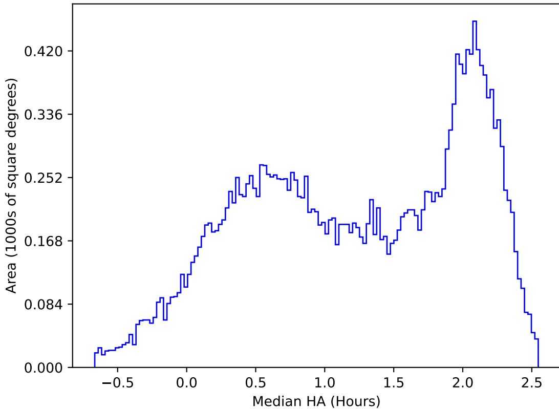
extra_ss_neo7_v3.4_10yrs All sky y band: Median HA
