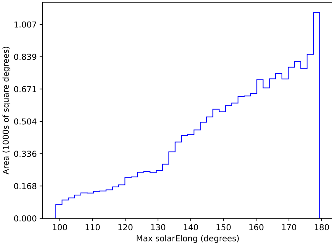
extra_ss_neo7_v3.4_10yrs WFD z band: Max solarElong
