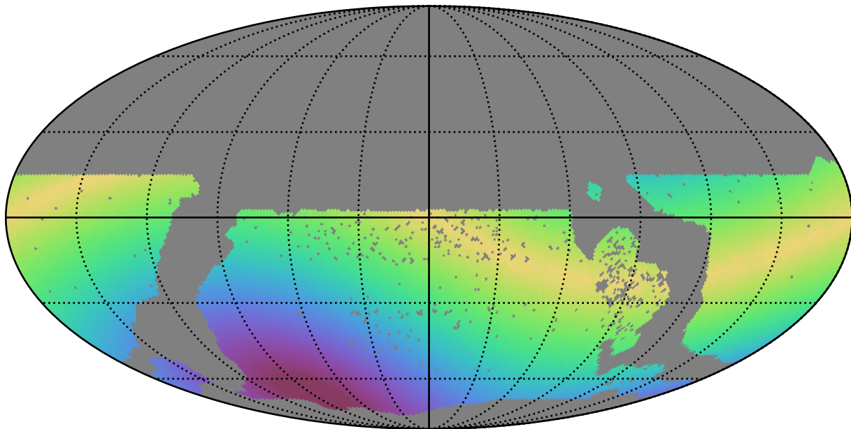
extra_ss_neo7_v3.4_10yrs WFD y band: Max solarElong
