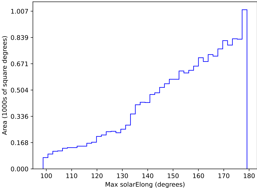
extra_ss_neo7_v3.4_10yrs WFD y band: Max solarElong
