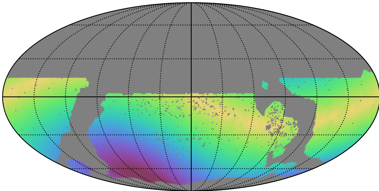
extra_ss_neo7_v3.4_10yrs WFD u band: Max solarElong
