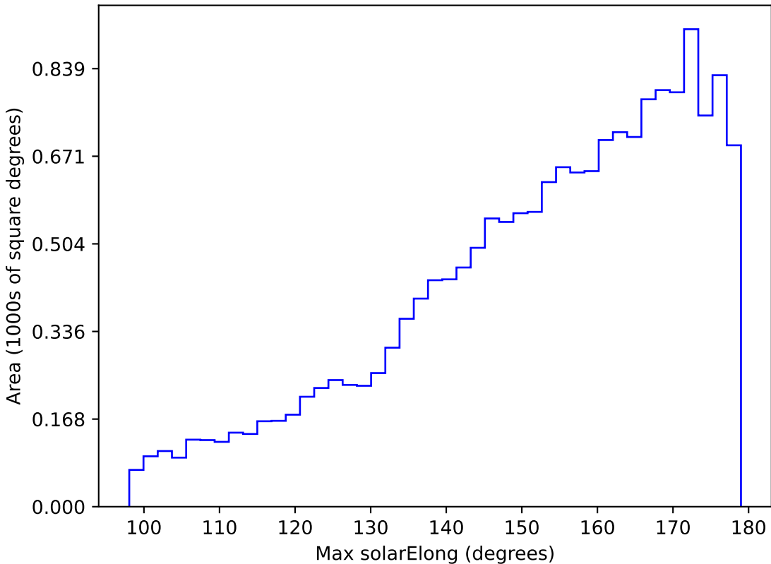
extra_ss_neo7_v3.4_10yrs WFD u band: Max solarElong
