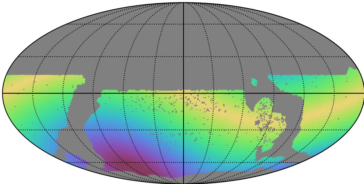
extra_ss_neo7_v3.4_10yrs WFD r band: Max solarElong
