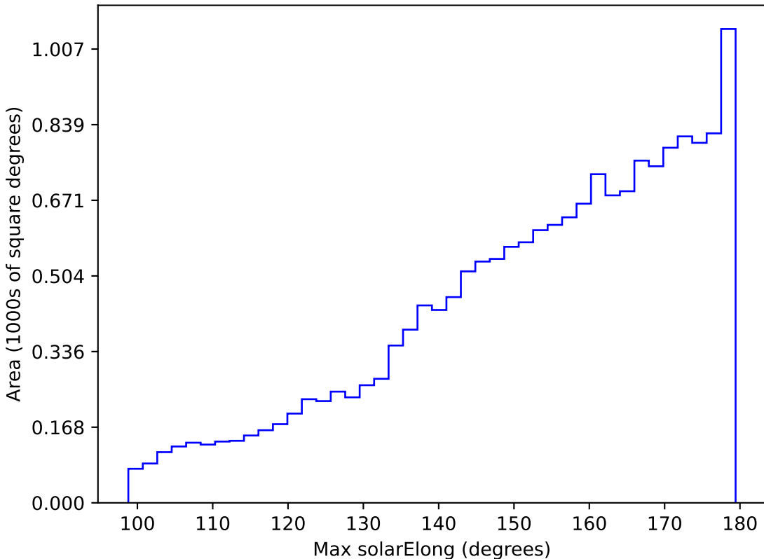
extra_ss_neo7_v3.4_10yrs WFD r band: Max solarElong
