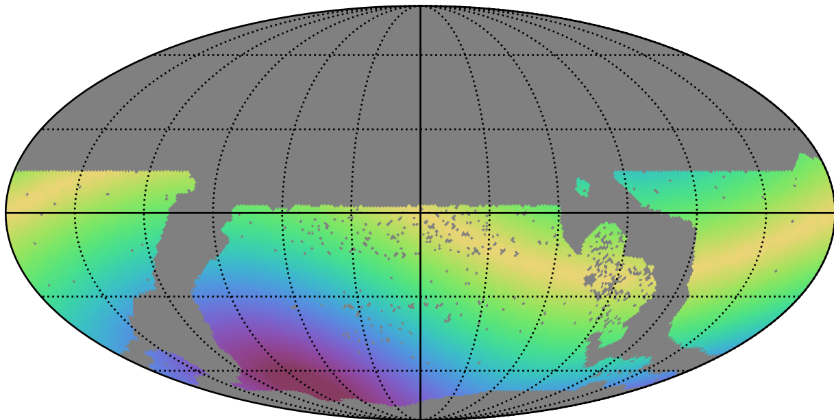
extra_ss_neo7_v3.4_10yrs WFD i band: Max solarElong
