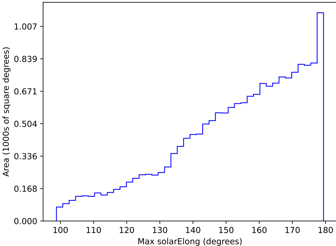
extra_ss_neo7_v3.4_10yrs WFD i band: Max solarElong
