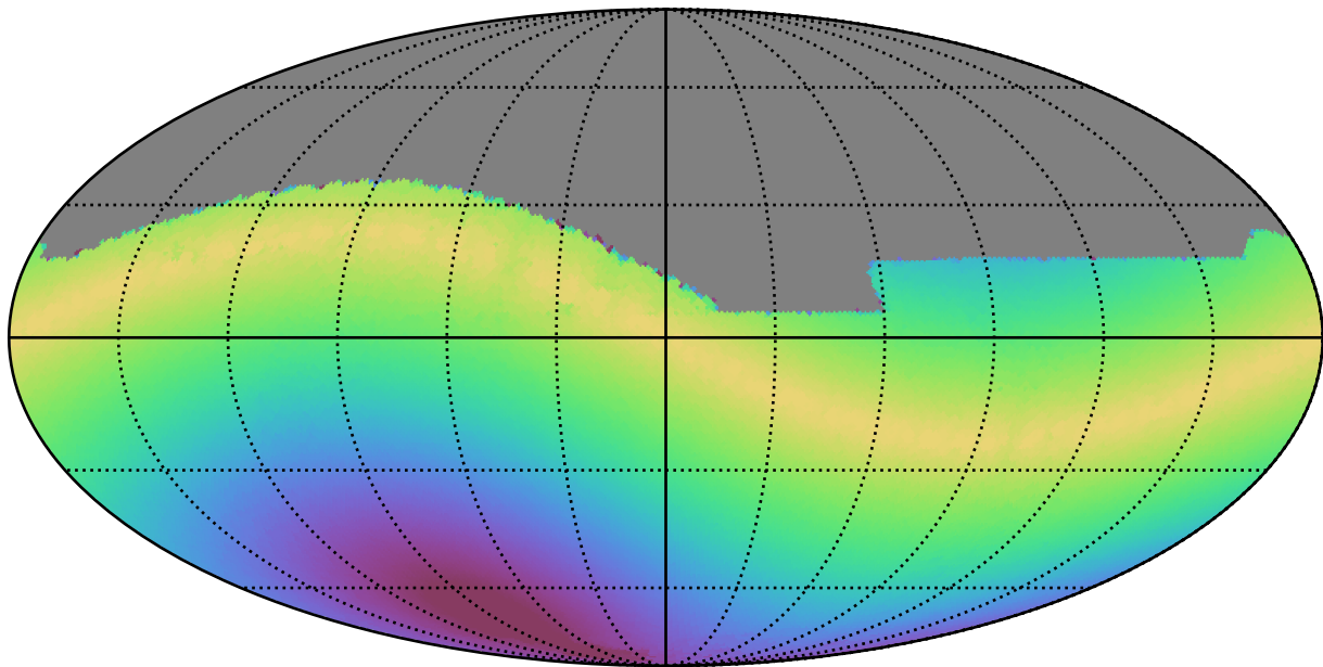
extra_ss_neo7_v3.4_10yrs All sky z band: Max solarElong
