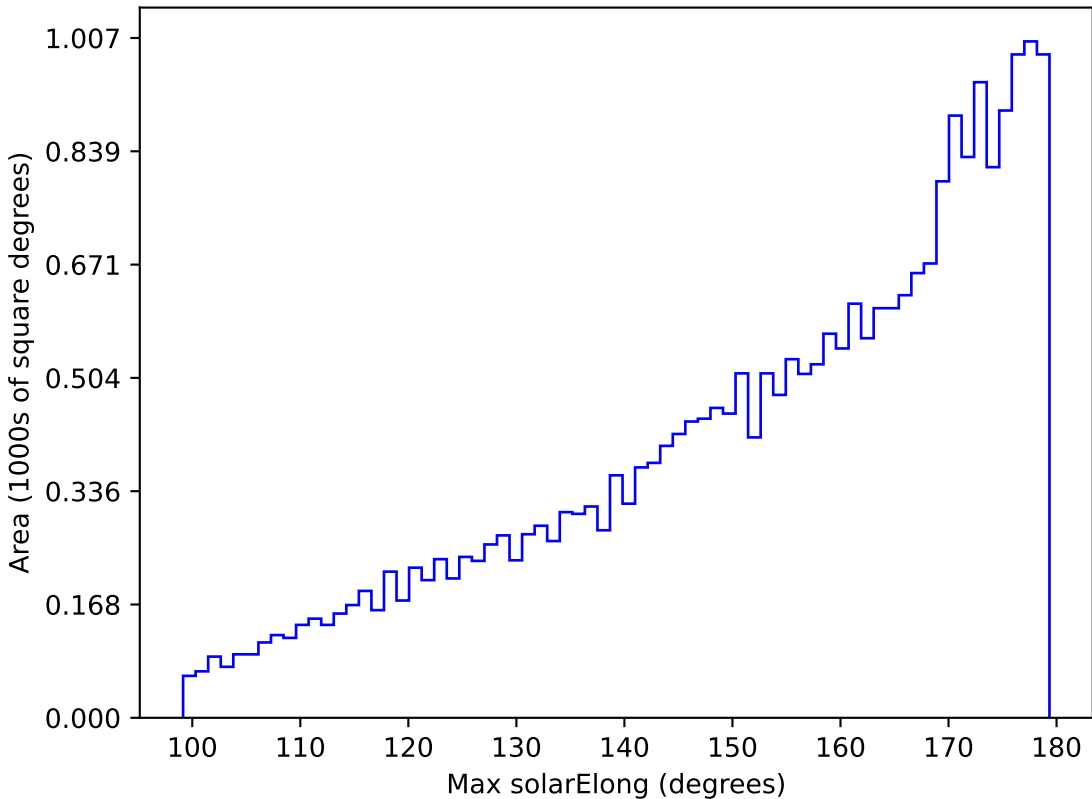
extra_ss_neo7_v3.4_10yrs All sky z band: Max solarElong
