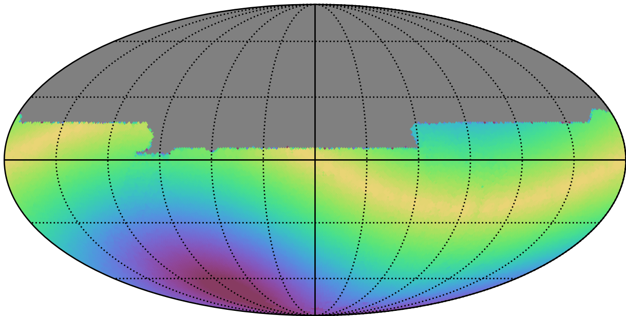
extra_ss_neo7_v3.4_10yrs All sky y band: Max solarElong
