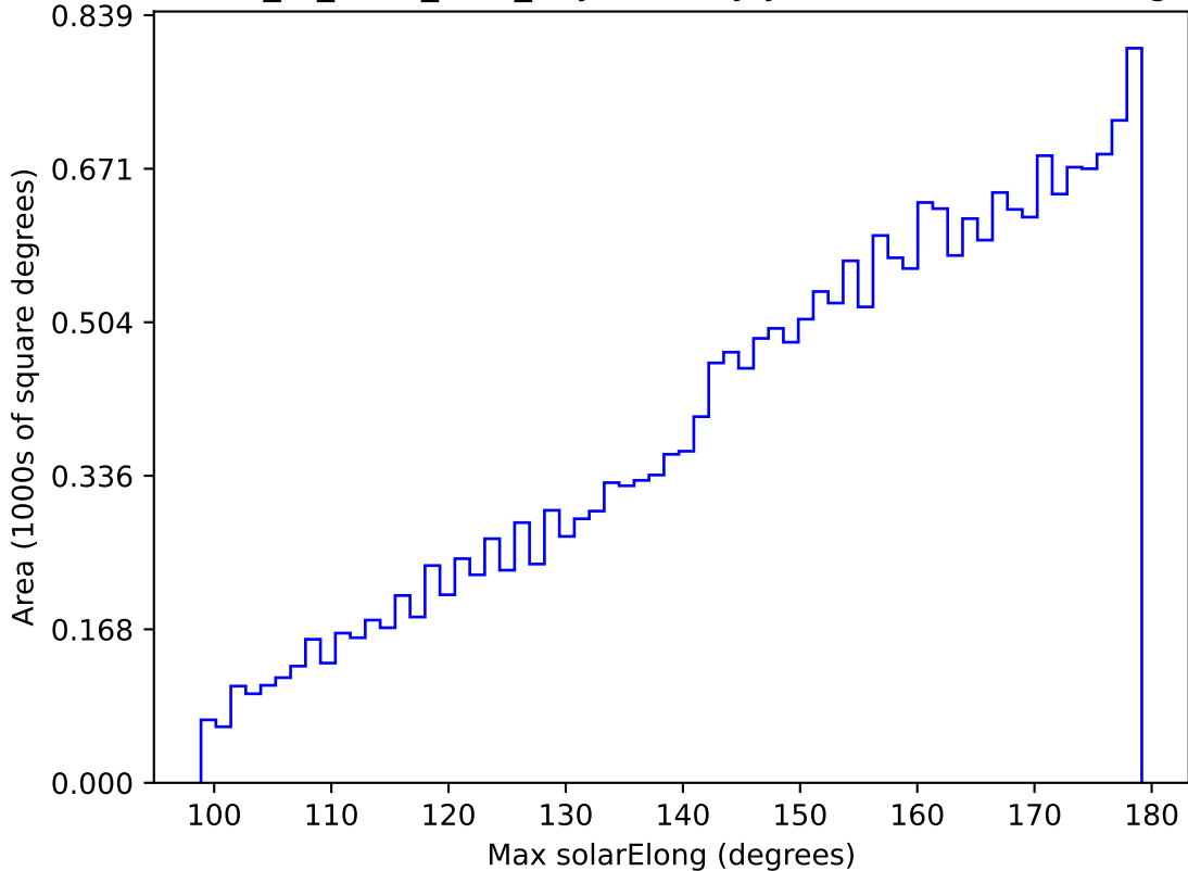
extra_ss_neo7_v3.4_10yrs All sky y band: Max solarElong
