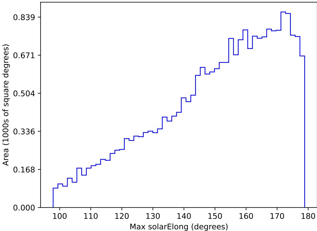
extra_ss_neo7_v3.4_10yrs All sky u band: Max solarElong
