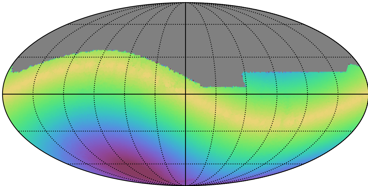
extra_ss_neo7_v3.4_10yrs All sky r band: Max solarElong
