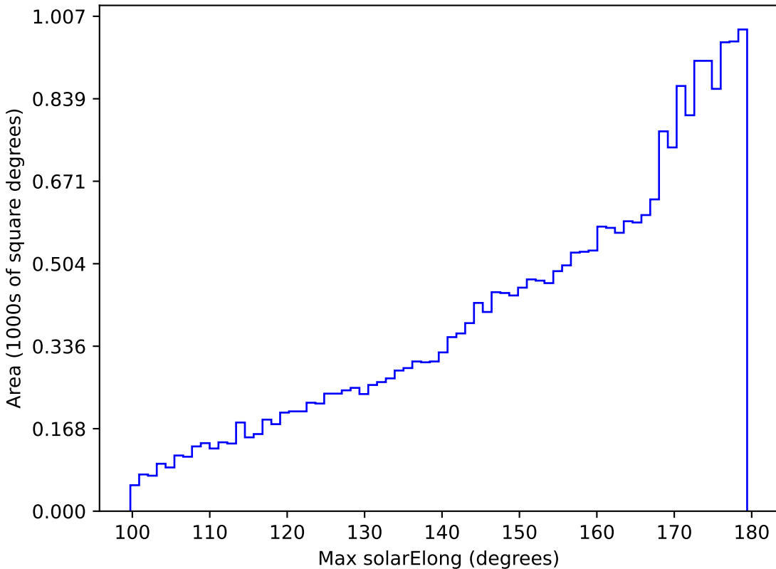
extra_ss_neo7_v3.4_10yrs All sky r band: Max solarElong
