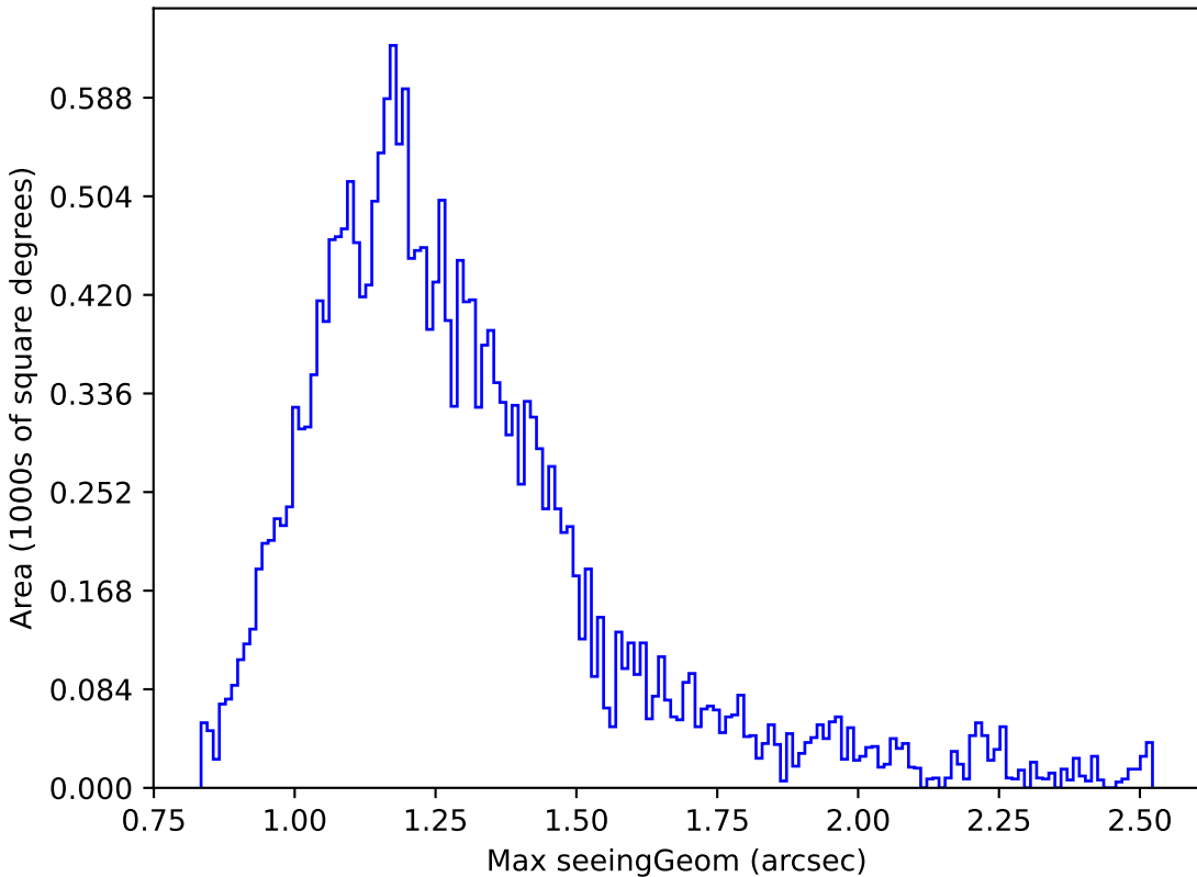
extra_ss_neo7_v3.4_10yrs Yr 1 y band: Max seeingGeom
