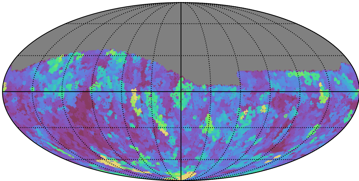
extra_ss_neo7_v3.4_10yrs Yr 1 i band: Max seeingGeom
