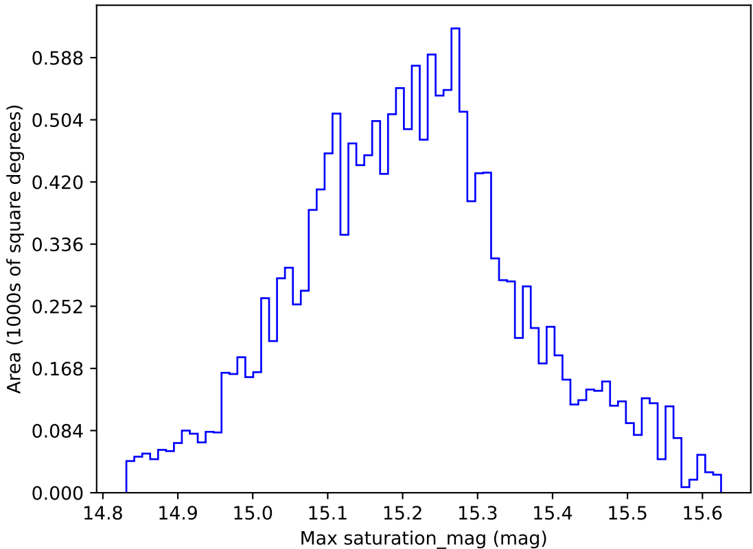
extra_ss_neo7_v3.4_10yrs WFD z band: Max saturation_mag
