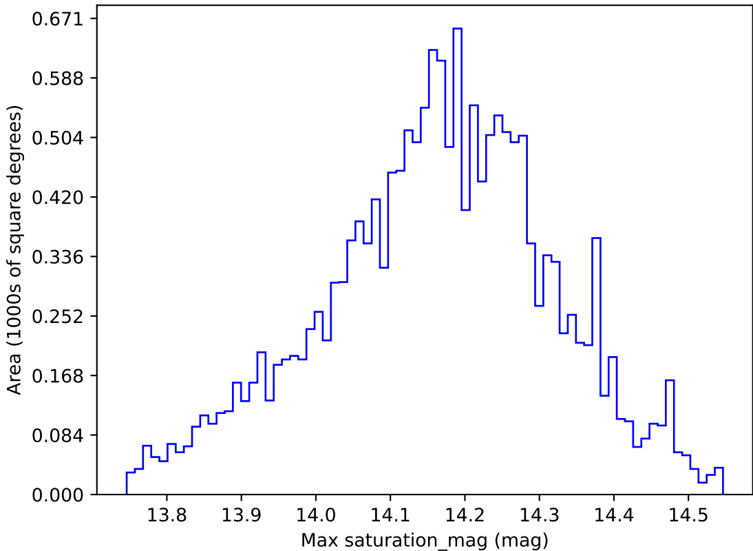
extra_ss_neo7_v3.4_10yrs WFD y band: Max saturation_mag
