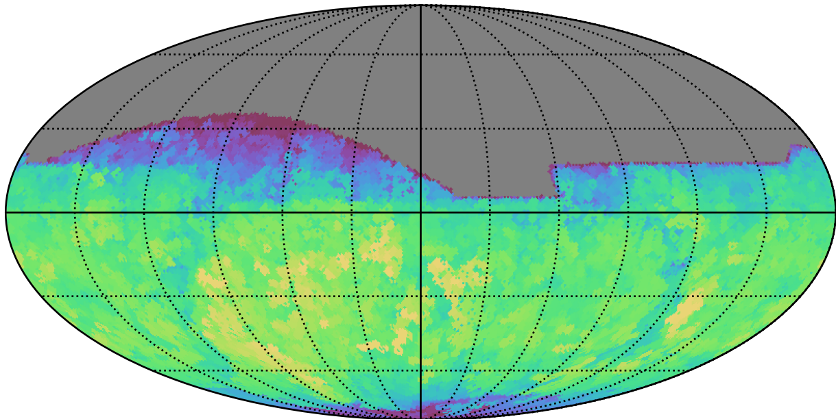
extra_ss_neo7_v3.4_10yrs All sky z band: Max saturation_mag
