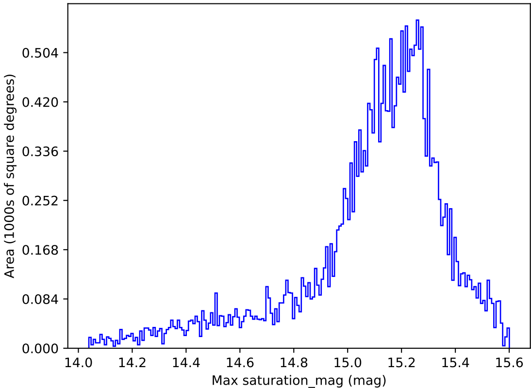
extra_ss_neo7_v3.4_10yrs All sky z band: Max saturation_mag
