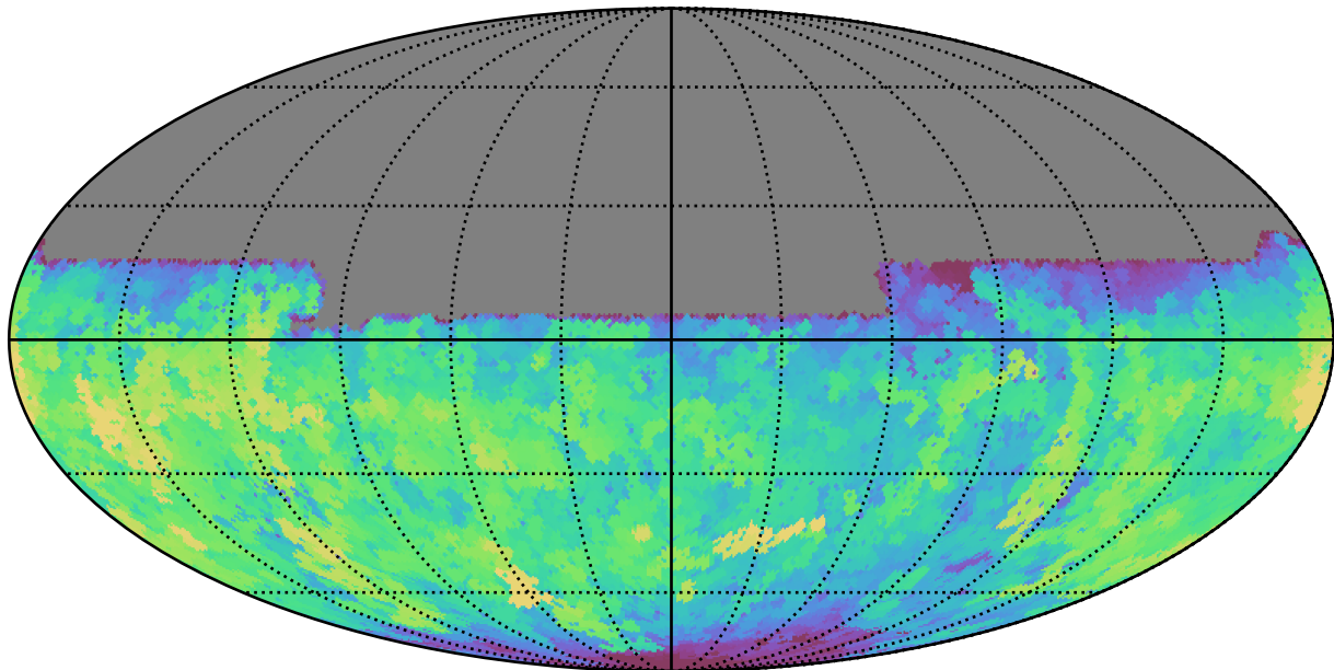
extra_ss_neo7_v3.4_10yrs All sky u band: Max saturation_mag
