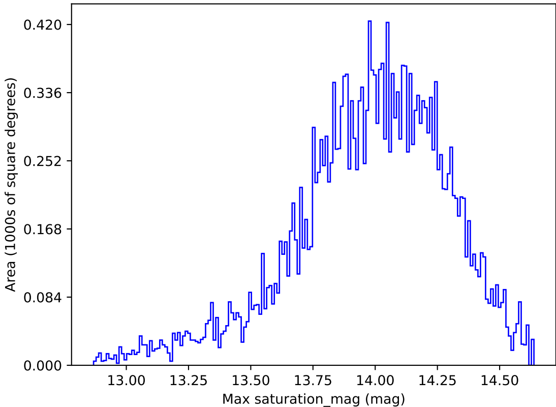
extra_ss_neo7_v3.4_10yrs All sky u band: Max saturation_mag
