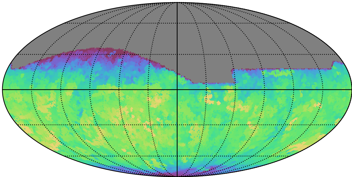
extra_ss_neo7_v3.4_10yrs All sky i band: Max saturation_mag
