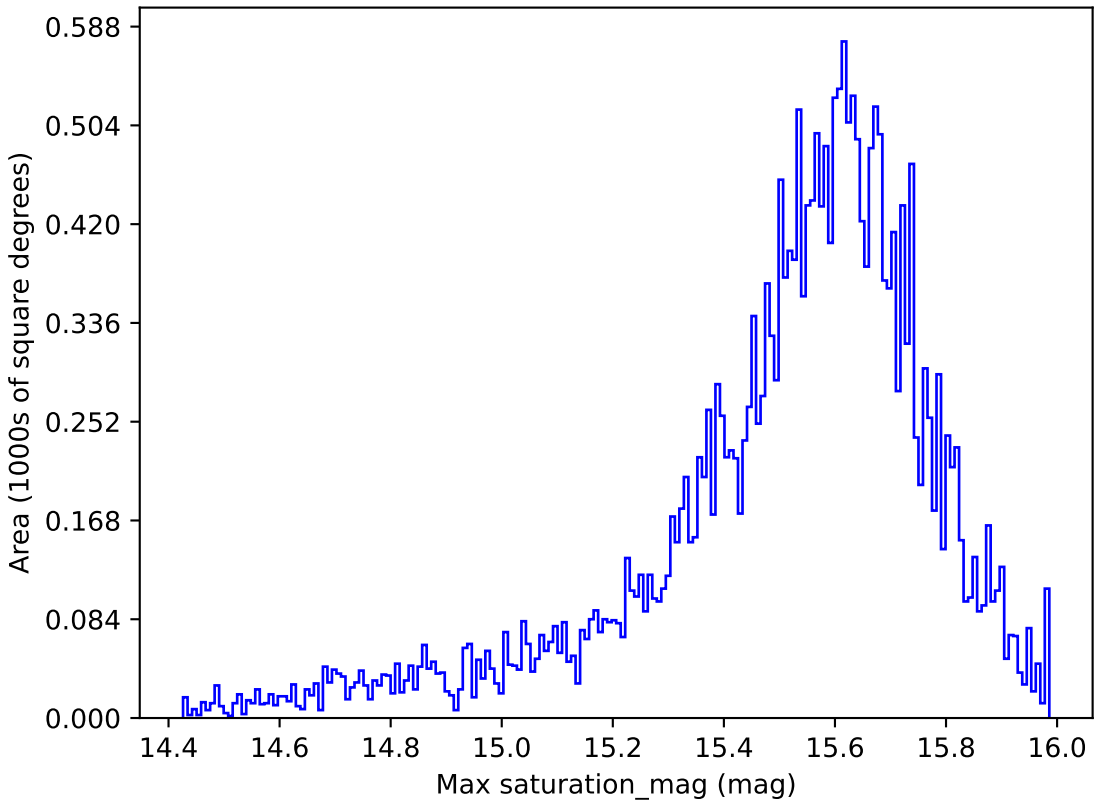
extra_ss_neo7_v3.4_10yrs All sky i band: Max saturation_mag
