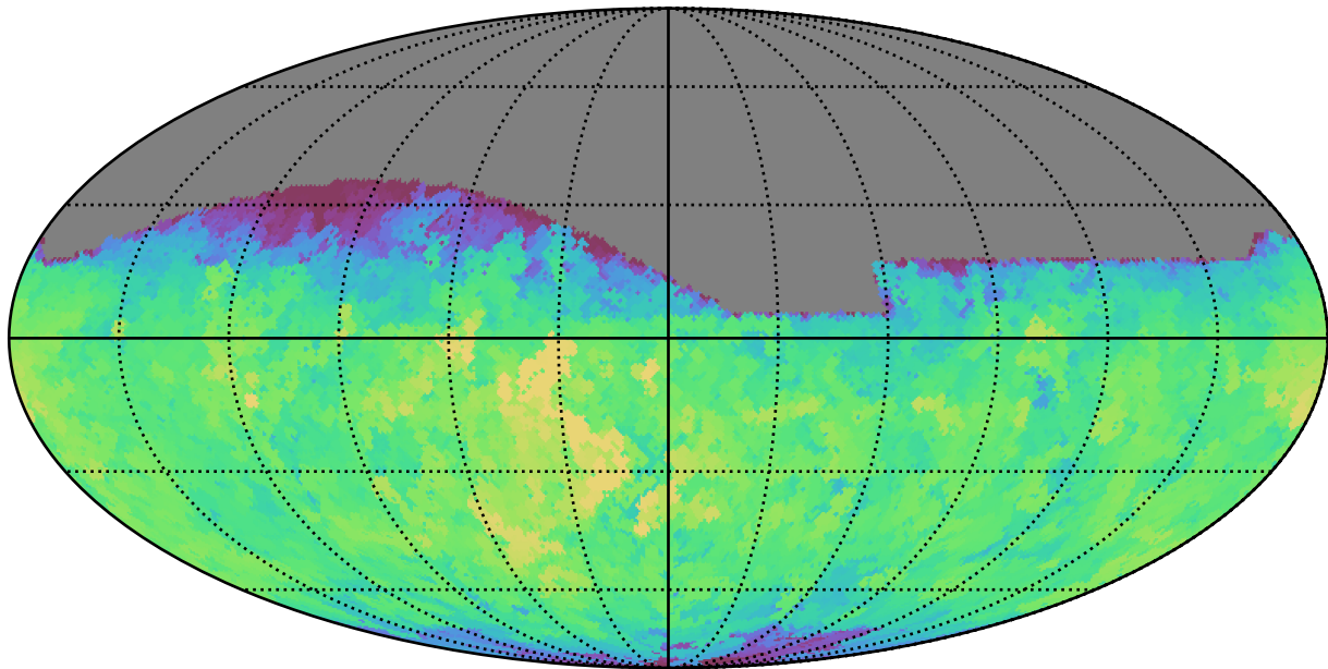
extra_ss_neo7_v3.4_10yrs All sky g band: Max saturation_mag
