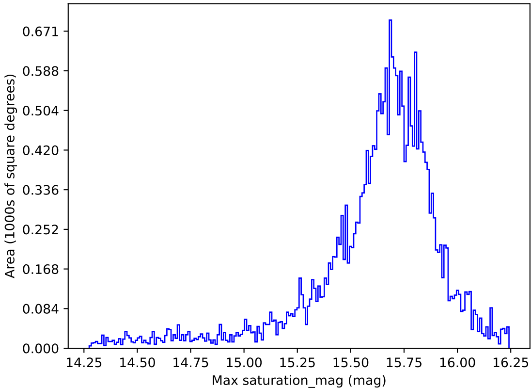
extra_ss_neo7_v3.4_10yrs All sky g band: Max saturation_mag
