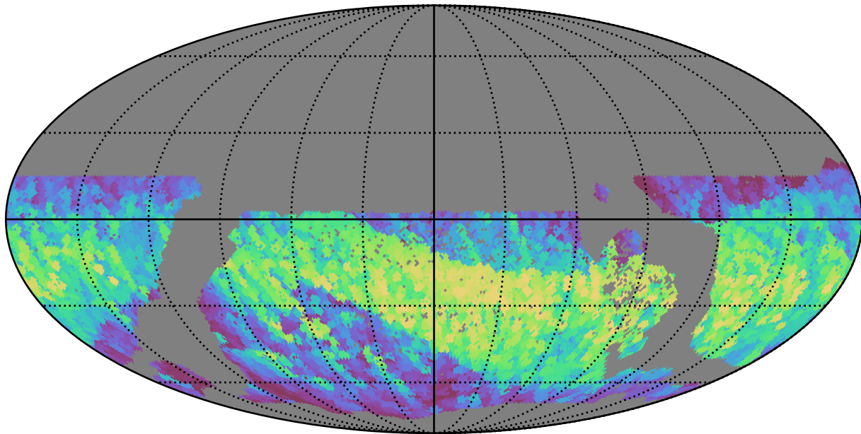
extra_ss_neo7_v3.4_10yrs WFD z band: Max normairmass
