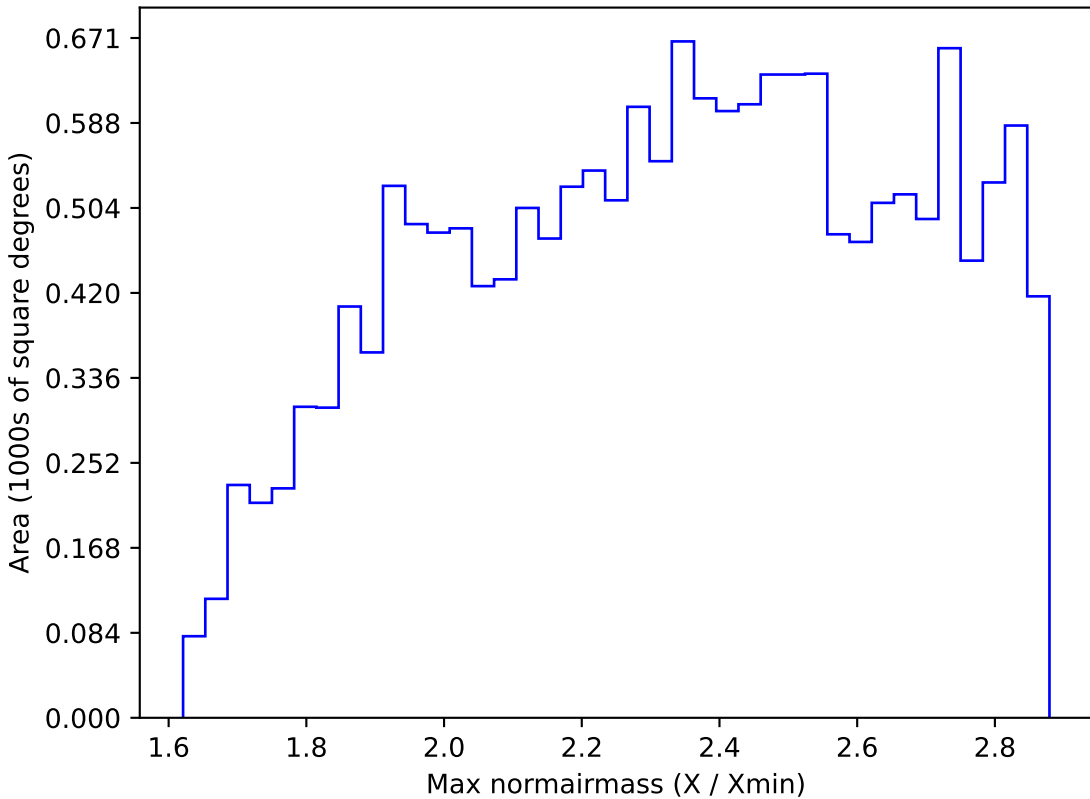
extra_ss_neo7_v3.4_10yrs WFD z band: Max normairmass
