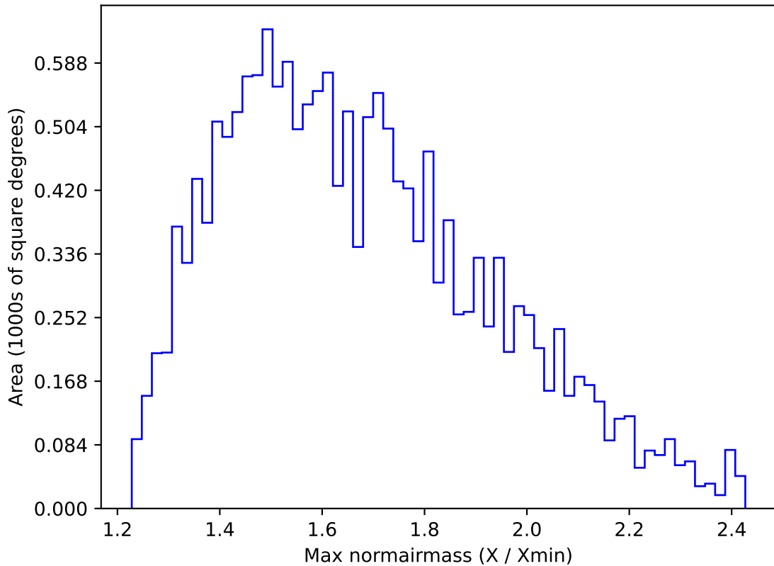
extra_ss_neo7_v3.4_10yrs WFD u band: Max normairmass
