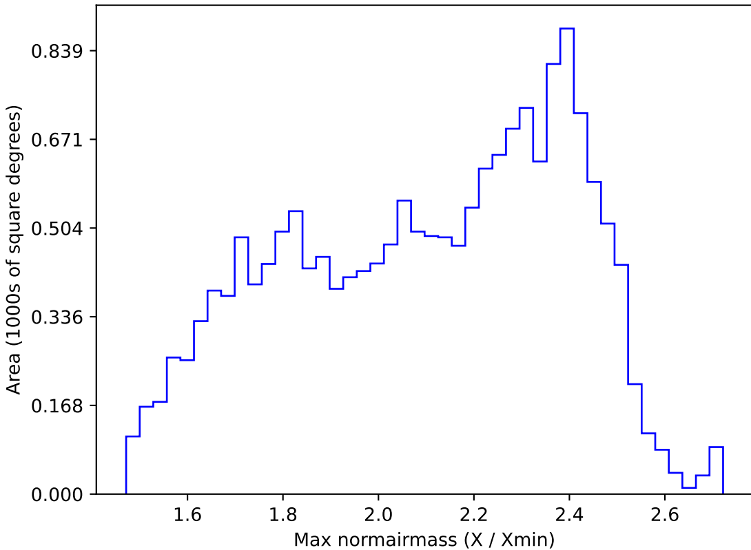
extra_ss_neo7_v3.4_10yrs WFD r band: Max normairmass
