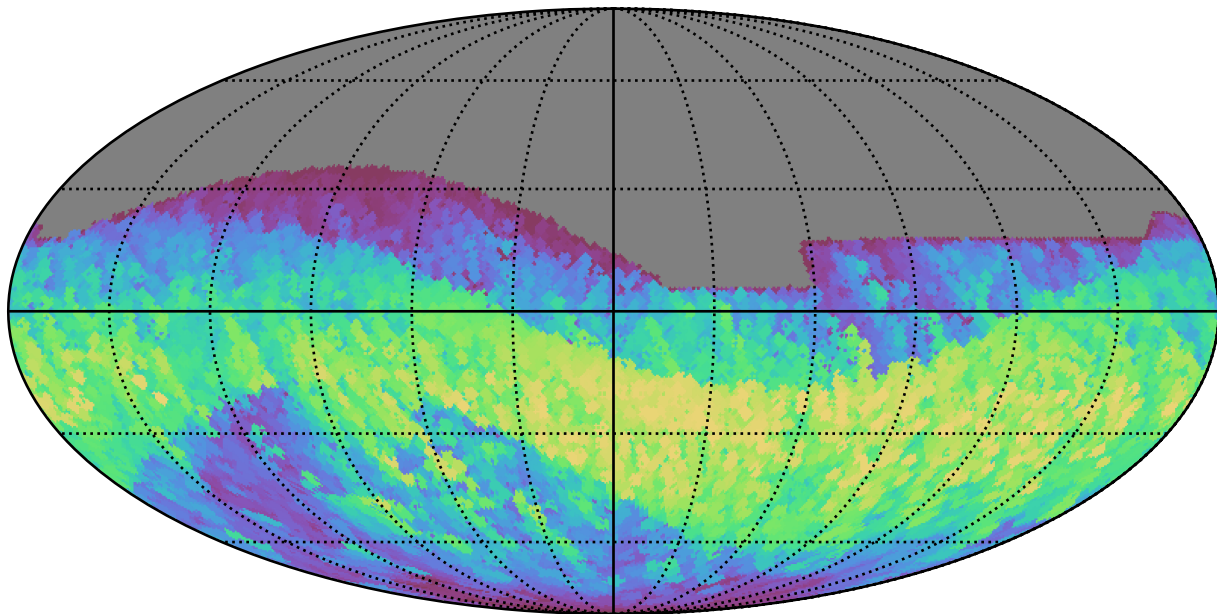
extra_ss_neo7_v3.4_10yrs All sky z band: Max normairmass
