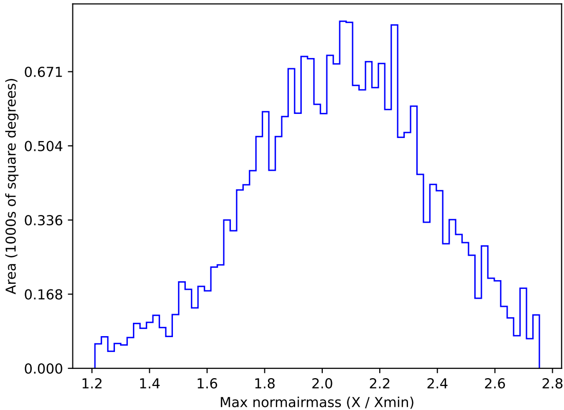
extra_ss_neo7_v3.4_10yrs All sky y band: Max normairmass
