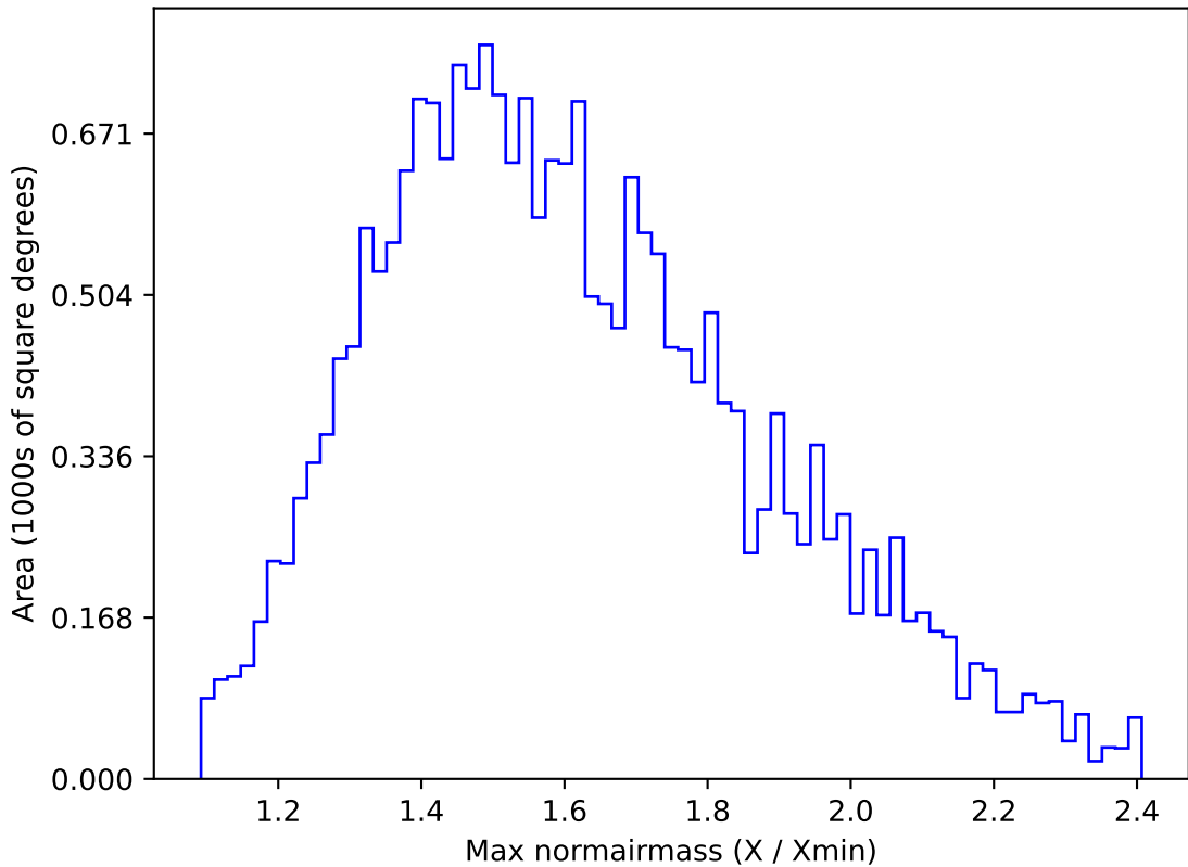
extra_ss_neo7_v3.4_10yrs All sky u band: Max normairmass
