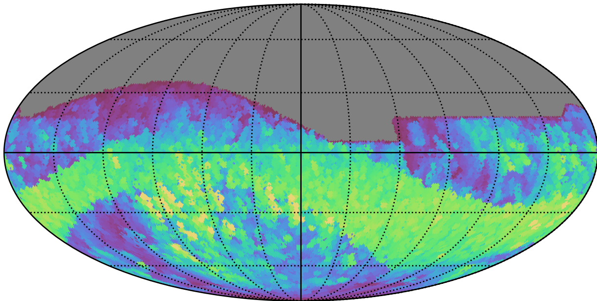
extra_ss_neo7_v3.4_10yrs All sky r band: Max normairmass
