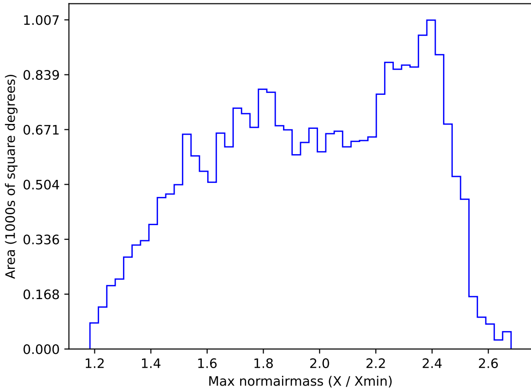
extra_ss_neo7_v3.4_10yrs All sky r band: Max normairmass
