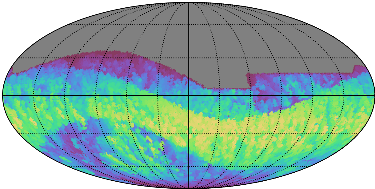
extra_ss_neo7_v3.4_10yrs All sky i band: Max normairmass
