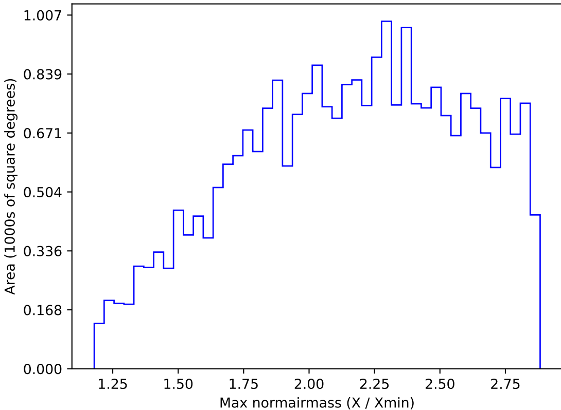
extra_ss_neo7_v3.4_10yrs All sky i band: Max normairmass
