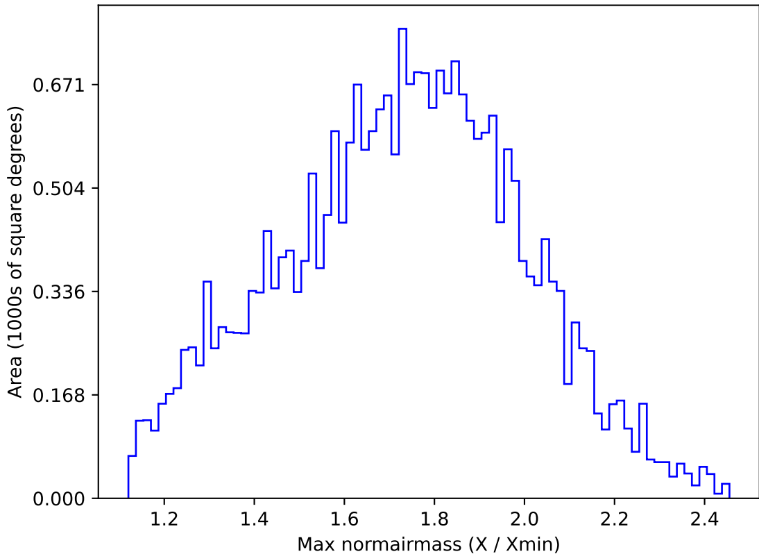
extra_ss_neo7_v3.4_10yrs All sky g band: Max normairmass
