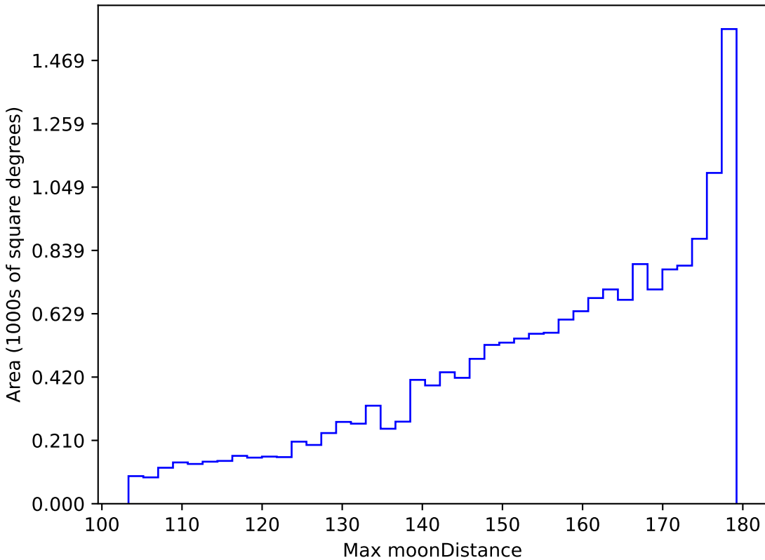
extra_ss_neo7_v3.4_10yrs WFD r band: Max moonDistance
