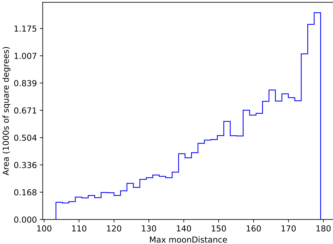
extra_ss_neo7_v3.4_10yrs WFD i band: Max moonDistance
